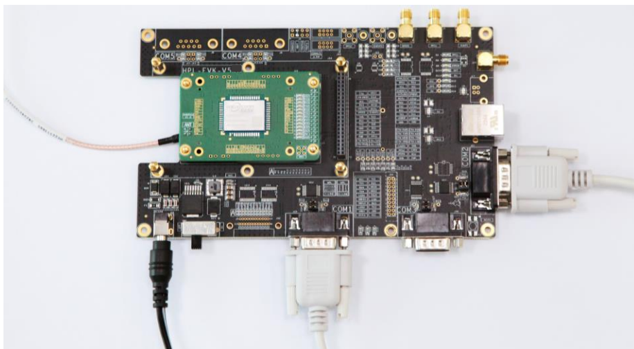
图 3-1 安装与连接
