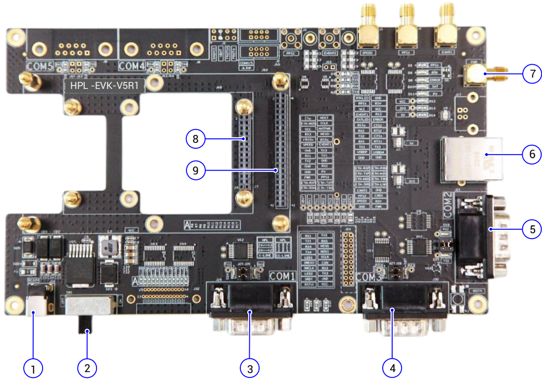
图 2-1 EVK 外观
